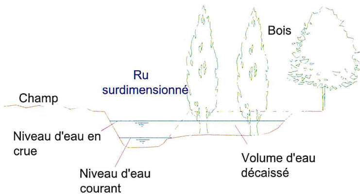
Coupe type d'une zone tampon
