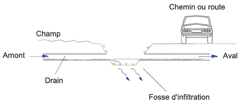
Coupe type d'un fossé en escalier
