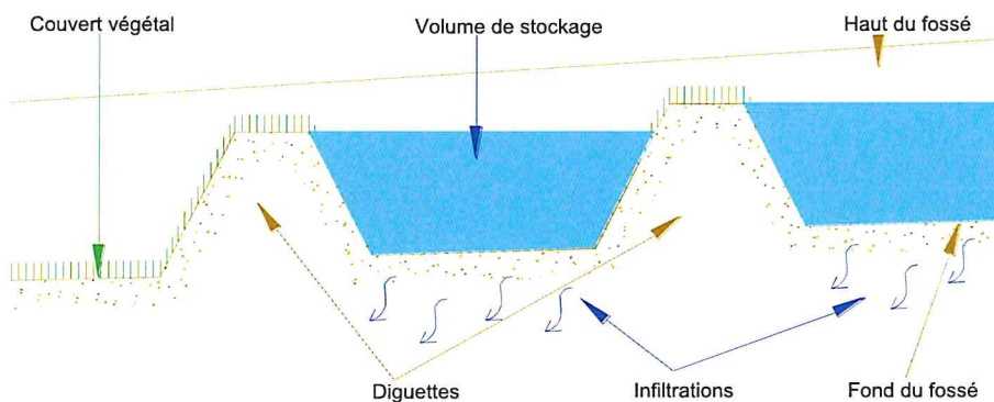
Coupe type d'un fossé en escalier
